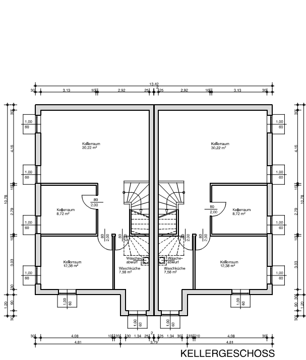
KELLERGESCHOSS
