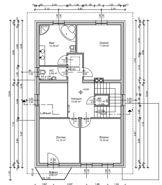
OBERGESCHOSS
