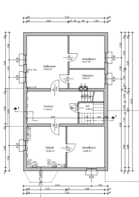
KELLERGESCHOSS
