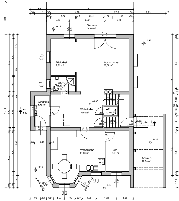
ERDGESCHOSS
